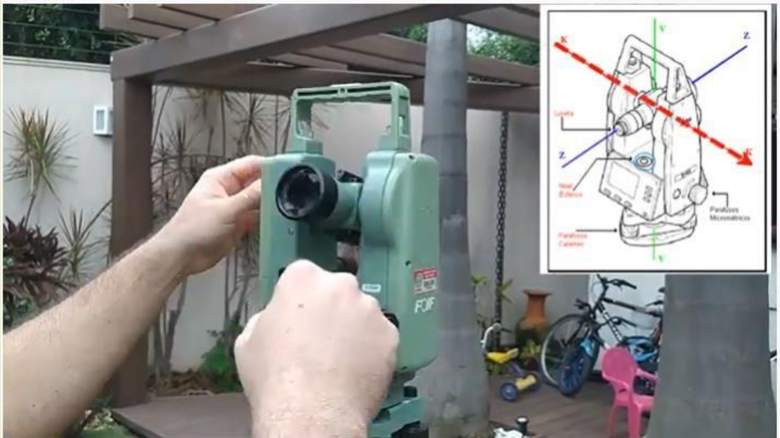
Topografia na prática - Aula 1: conhecendo os instrumentos | Prof. Edgar Demarqui
